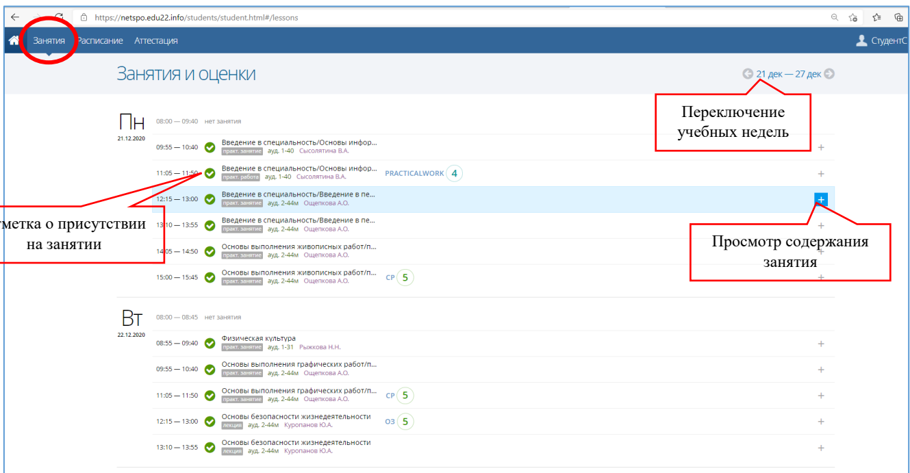
Рисунок 4 – Электронный дневник
